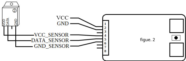
Câblage du capteur DHT22
