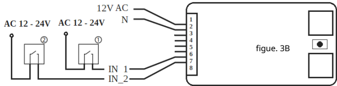
Câblage du capteur binaire (ampoule Reed)
