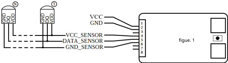
Câblage du capteur DS18B20
