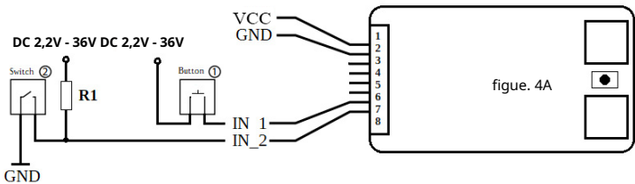
Câblage des boutons et interrupteurs
