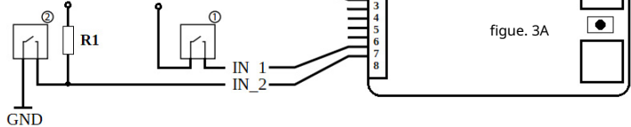
Câblage du capteur binaire (ampoule Reed)
