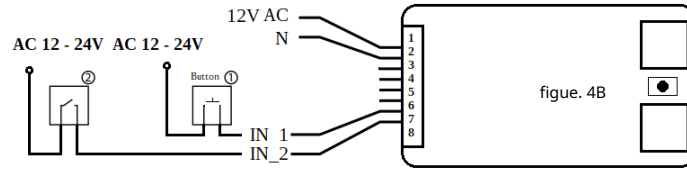
Câblage des boutons et interrupteurs
