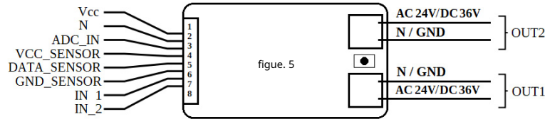
Câblage de charge
