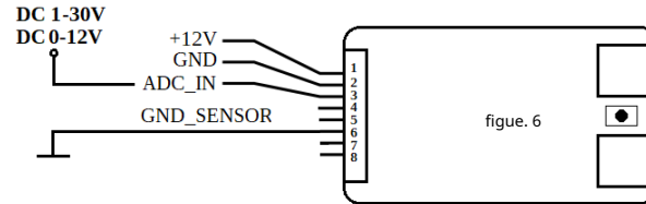
Câblage de l'ADC
